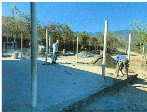
Foto 3: MEJORAMIENTO DE LOSA DE PISO EN PROCESO
