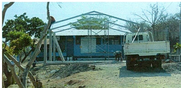
Foto 2: MEJORAMIENTO CON ESTRUCTURA TIPO PÓRICO E INSTALACIÓN DE LÁMINAS TROQUELADA CALIBRE 26, PARA AREA DE REUNIONES EN PROCESO.
